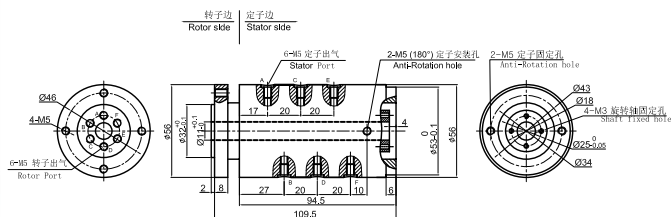
MQ600-01 尺寸图
