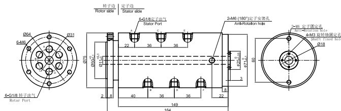
MQ600-02 尺寸图
