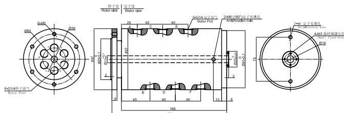
MQ600-03 尺寸图
