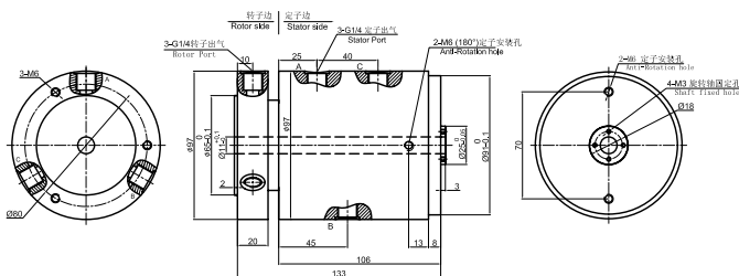
MQ300F-03 尺寸图
