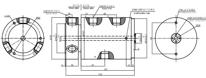
MQ300F-05 尺寸图
