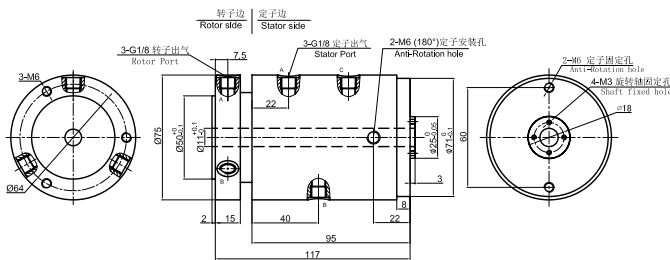
MQ300F-02 尺寸图
