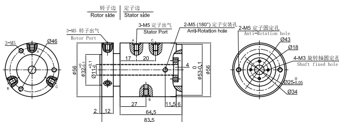
MQ300F-01 尺寸图
