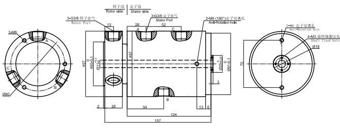
MQ300F-04 尺寸图
