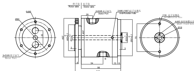
MQ200-05 尺寸图
