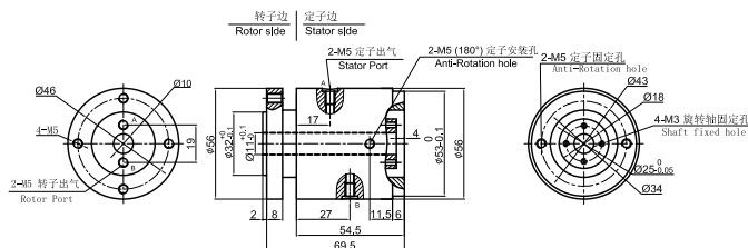
MQ200-01 尺寸图
