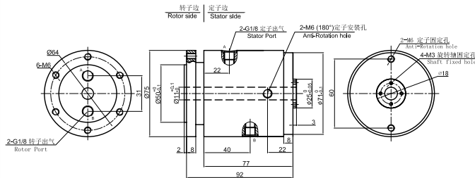
MQ200-03 尺寸图
