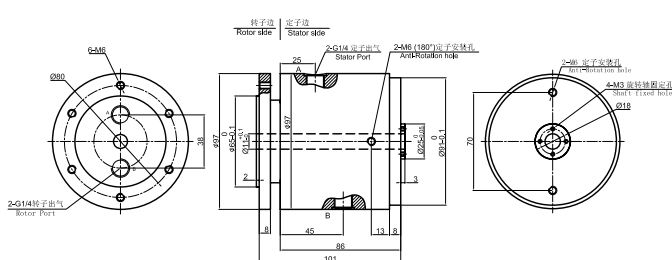
MQ200-03 尺寸图
