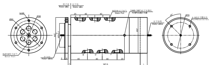
MAPH600S-03 尺寸图
