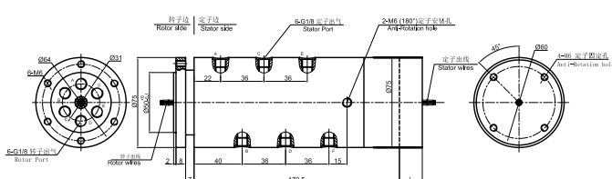
MAPH600S-03 尺寸图
