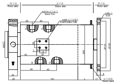
MAPH400W-03 尺寸图
