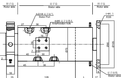
MAPH400W-03 尺寸图
