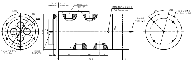
MAPH400S-05 尺寸图
