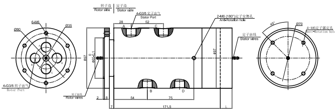
MAPH400S-05 尺寸图
