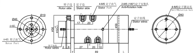
MAPH400S-01 尺寸图
