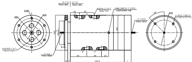
MAPH400S-03 尺寸图
