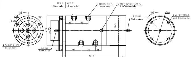
MAPH400S-03 尺寸图
