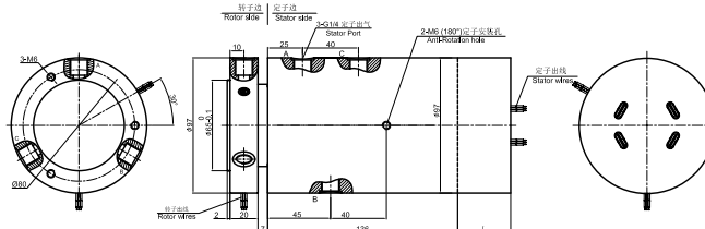
MAPH300F-03 尺寸图
