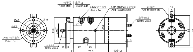
MAPH300-02 尺寸图
