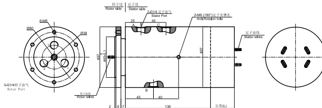
MAPH300-03 尺寸图
