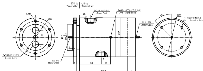
MAPH200S-05 尺寸图
