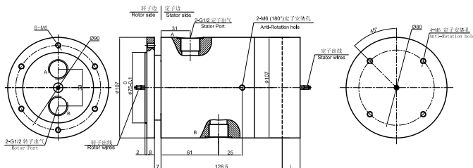
MAPH200S-05 尺寸图
